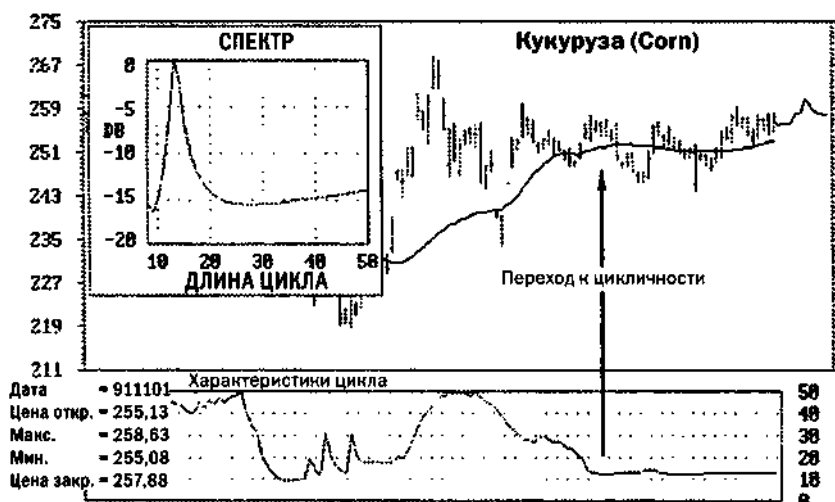
Рис. 5.6. Оценка циклов цен методом спектрального анализа максимальной энтропии (MESA)
