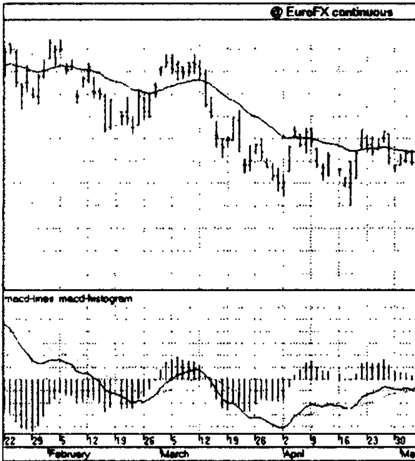
Рис. 5.9. Гистограмма MACD
