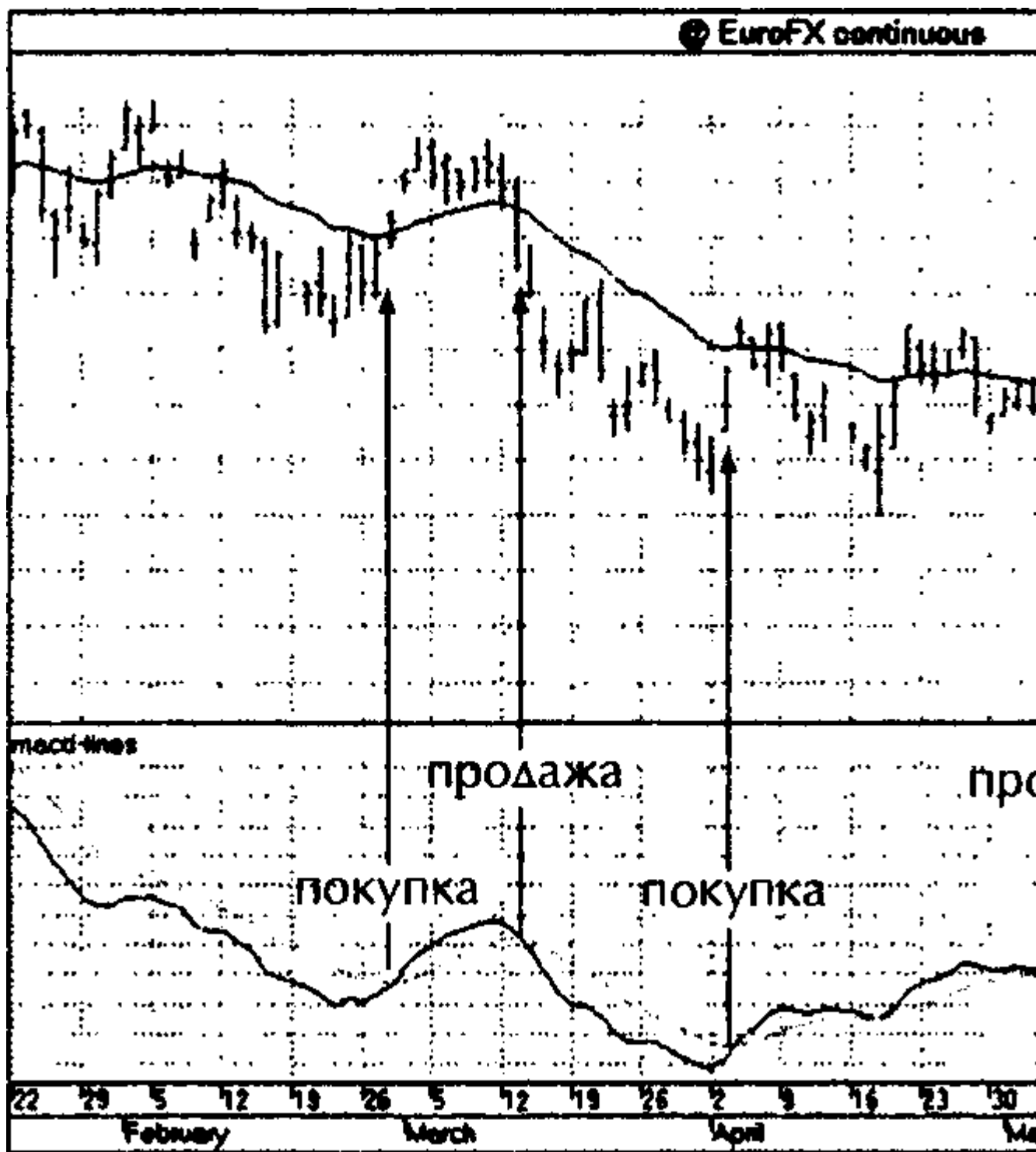
Рис. 5.8. Линии MACD
