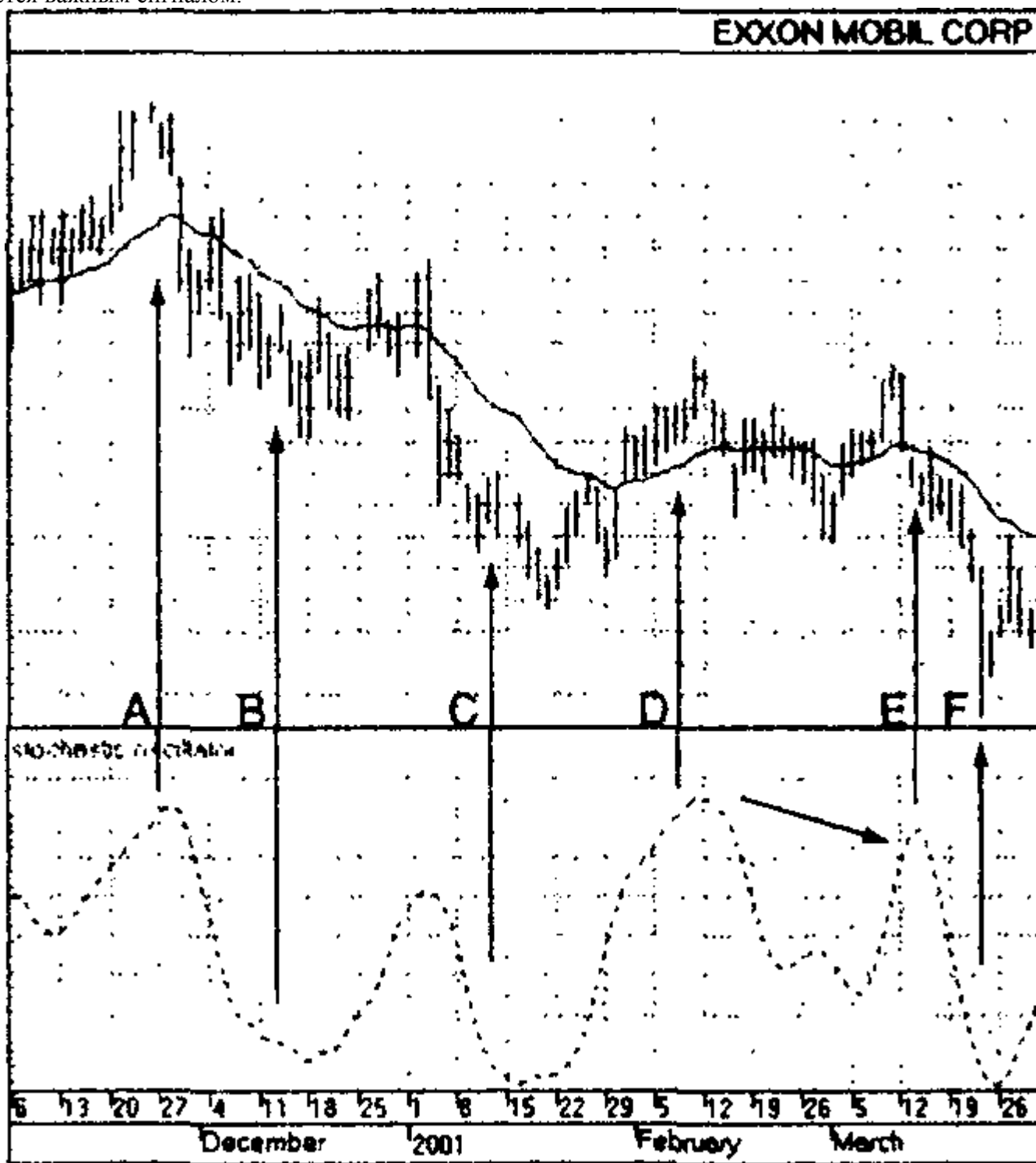
Рис. 5.14. Стохастический осциллятор
